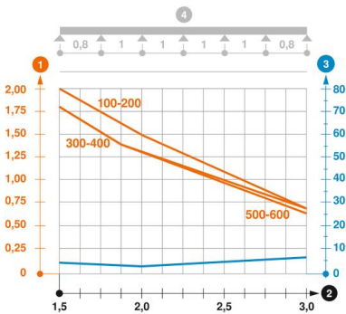
Diagrama de carga bandeja portacables MKSM 110
